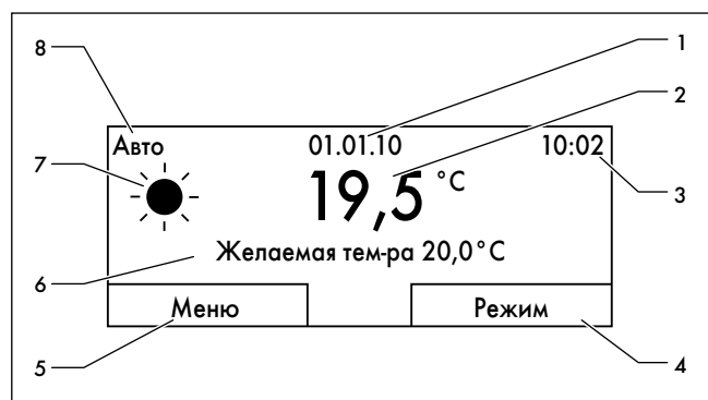
Рис. 3.3 Основная маска
